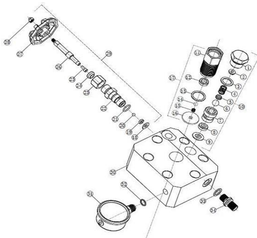
Сборка клапана
